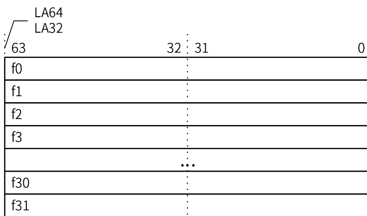
图 3-1 浮点寄存器
