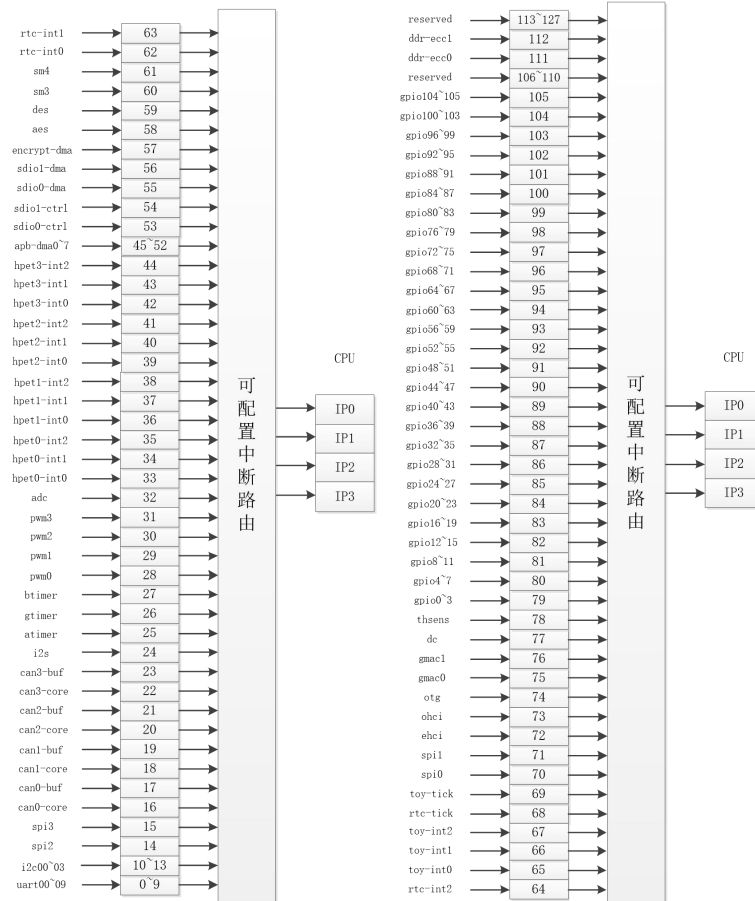
图3-3 龙芯 2K0301 扩展 IO 中断路由示意图
