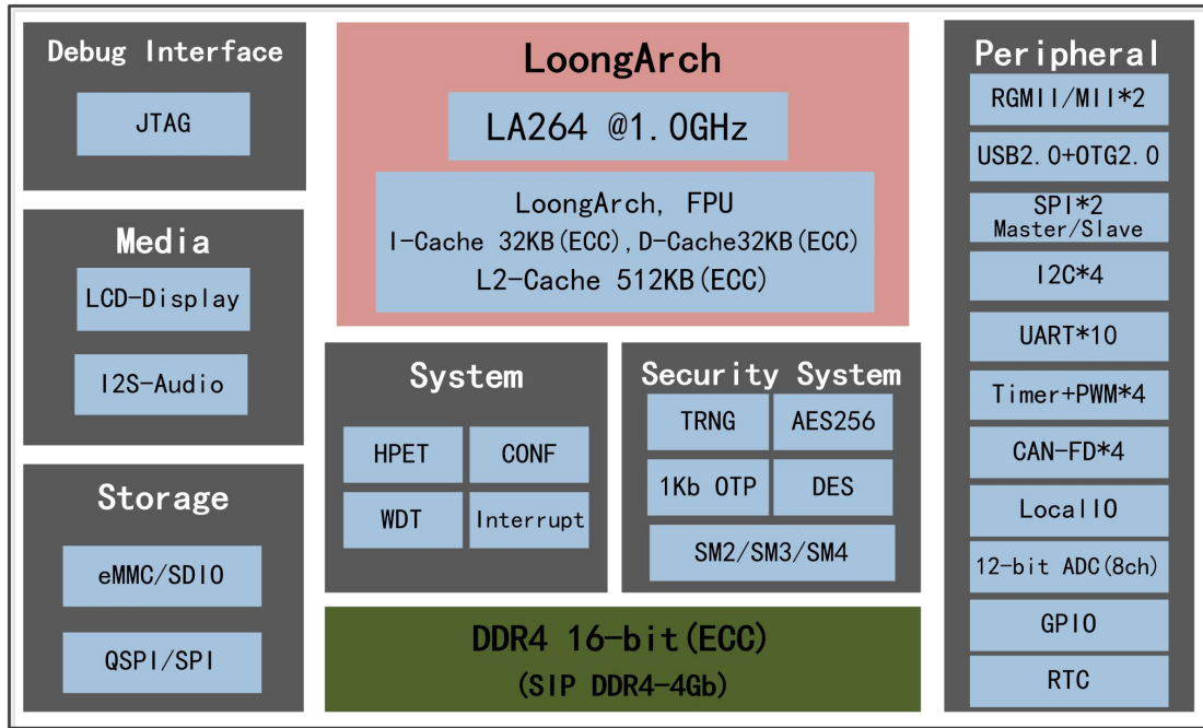
图1-1 龙芯 2K0301 芯片结构图
