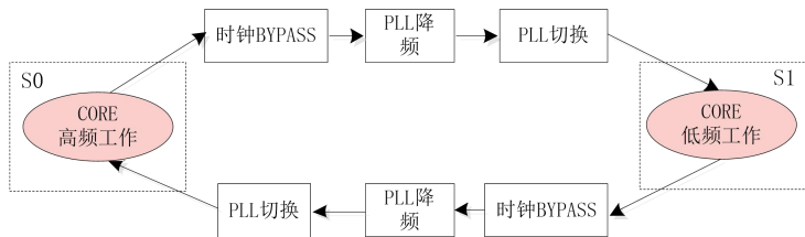
图26-1 处理器核 DFS 操作流程图
