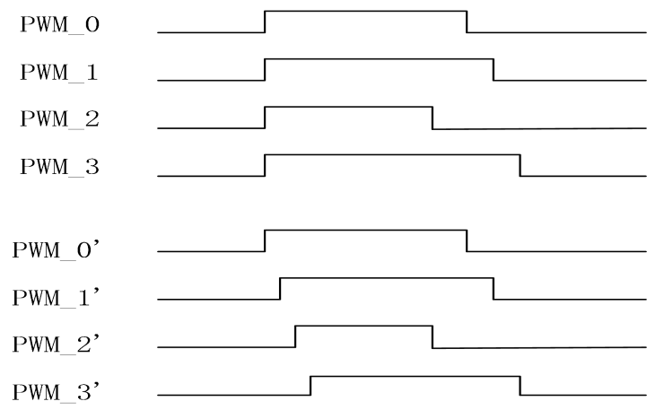
图21-1 防死区功能
