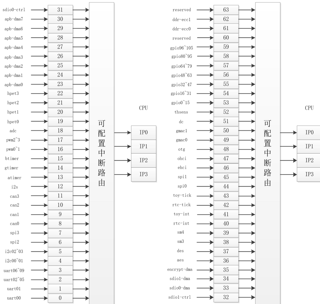
图3-2 龙芯 2K0301 传统中断路由示意图
