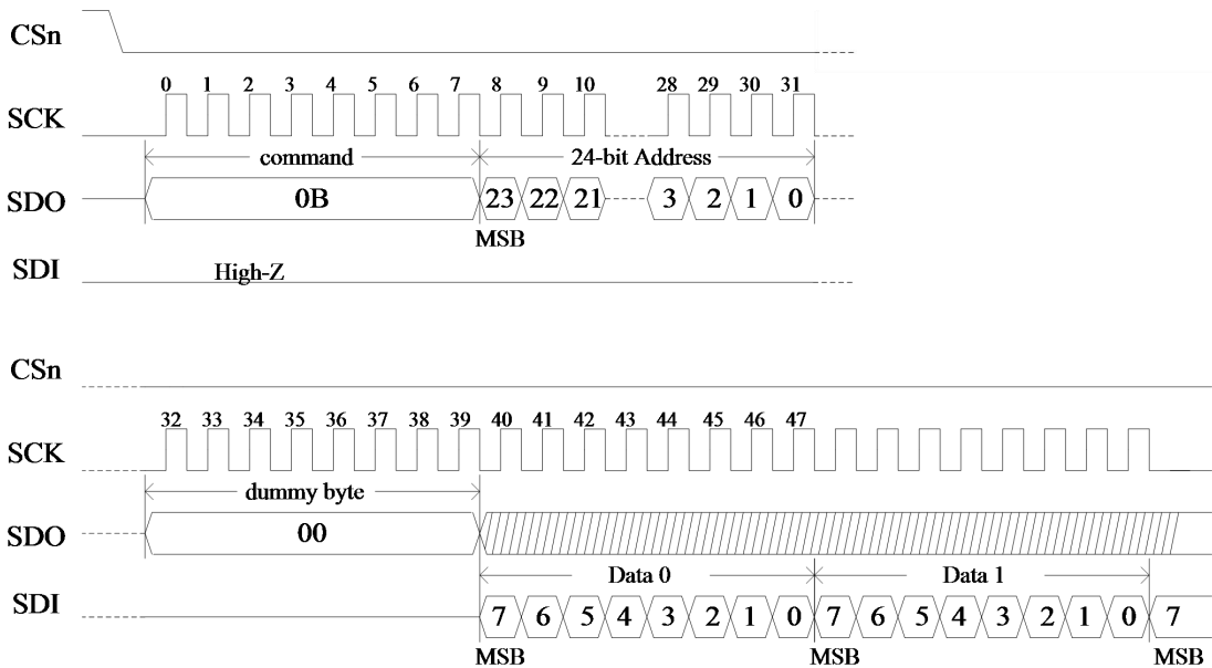
图9-4 SPI Flash 快速读时序
