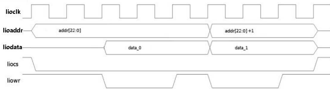
图13-2 LocalI/O 写时序
