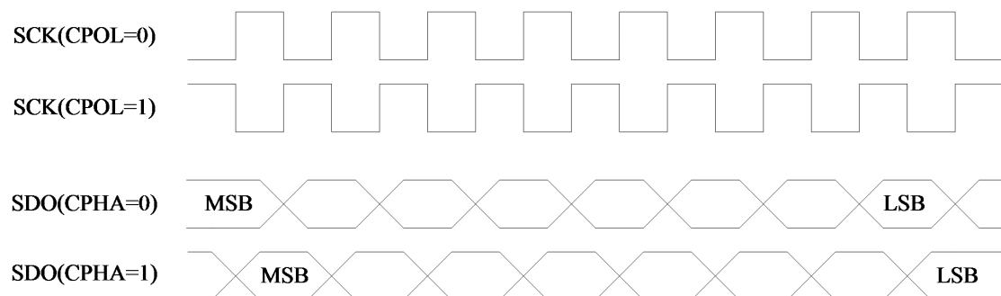
图9-2 SPI 主控制器接口时序
