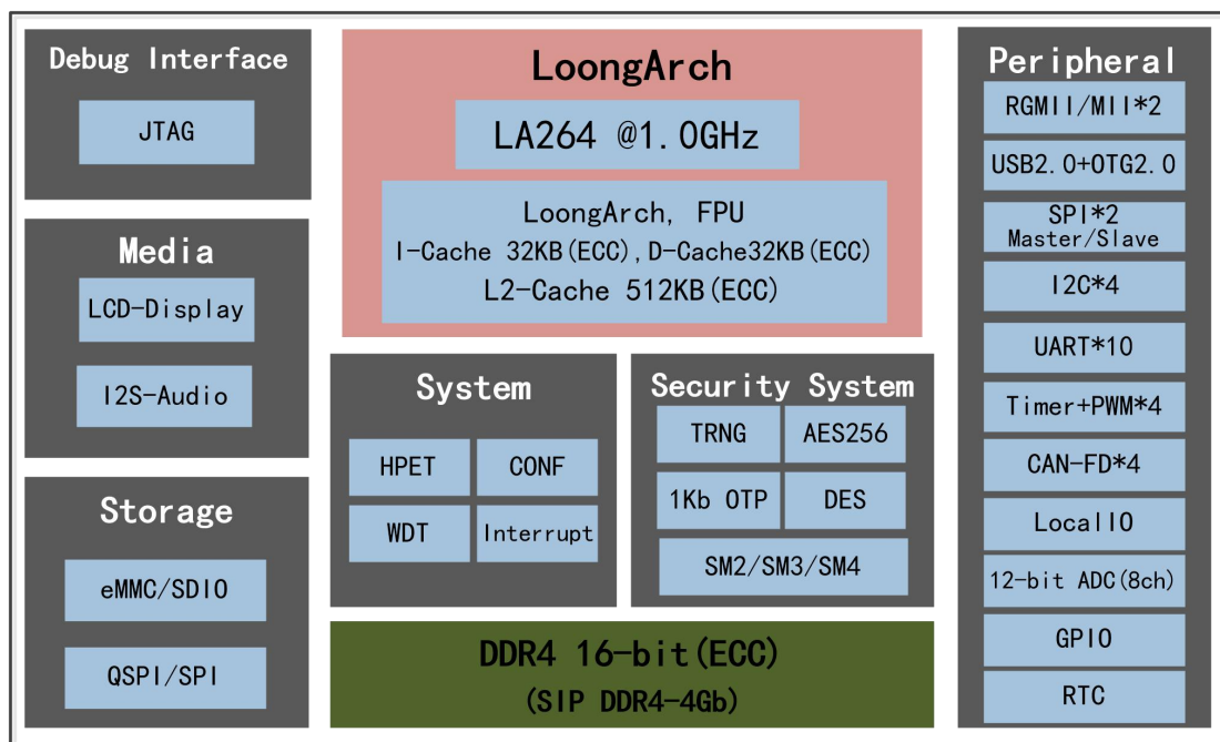
图 1.1 龙芯 2K0301 结构图
