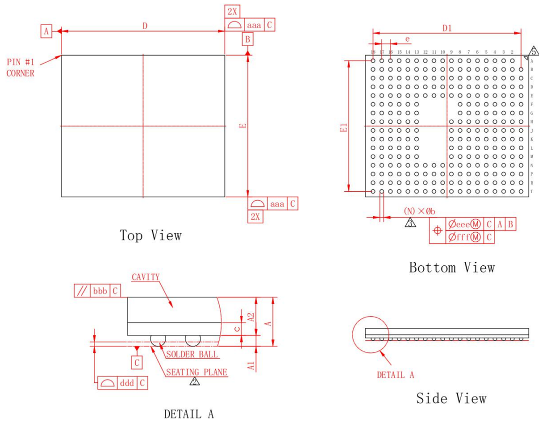
图 7.2 封装外形图
