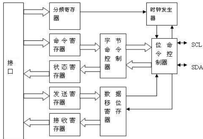
图 16- 1 I2C 主控制器结构
