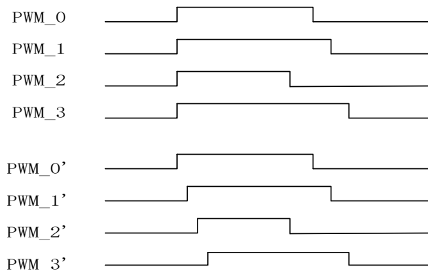
图 17- 1 防死区功能
