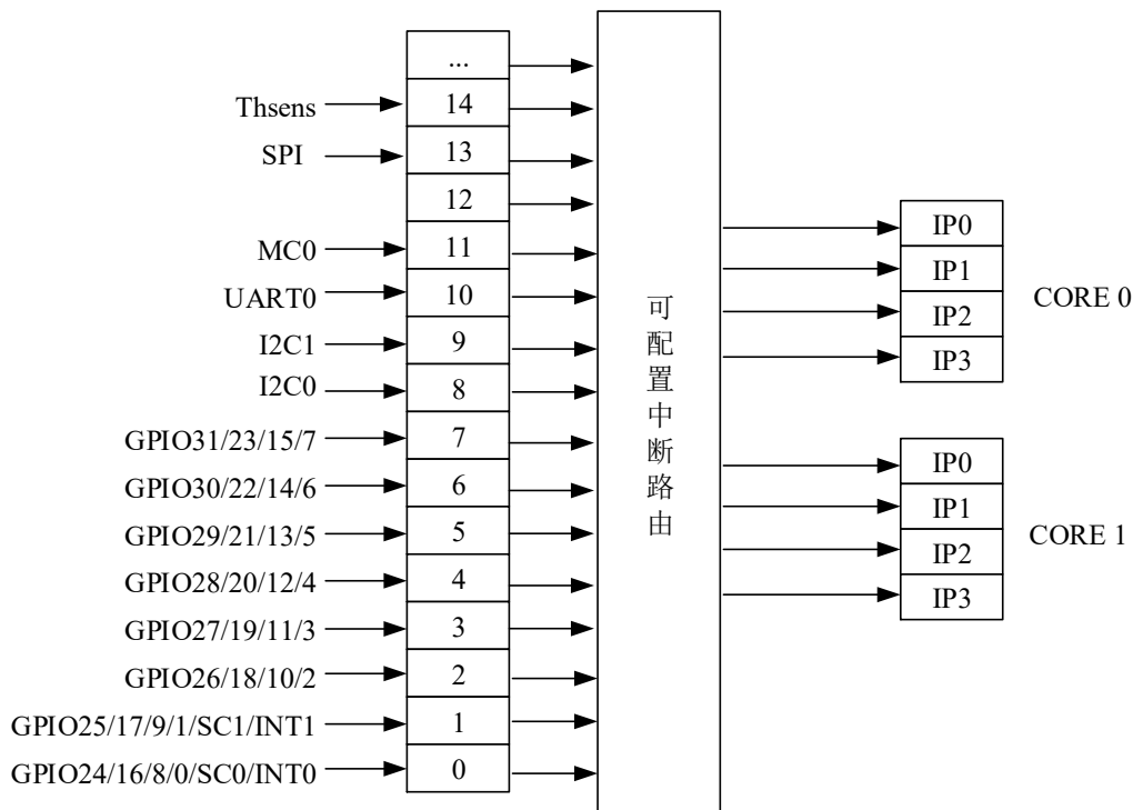
图 8- 2 龙芯 2K1500 处理器 NODE 中断路由示意图
