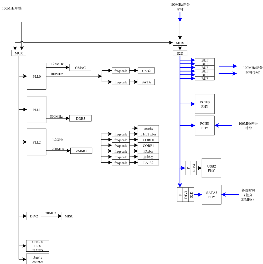
图 3- 1 芯片时钟结构图
