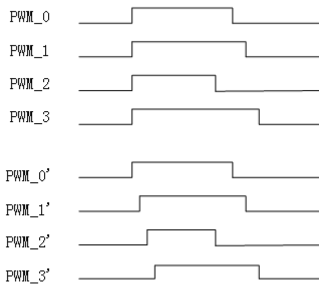
图 11-1. 防死区功能
