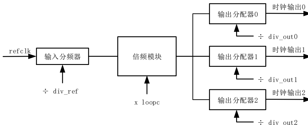
图 2-2. PLL 结构图
