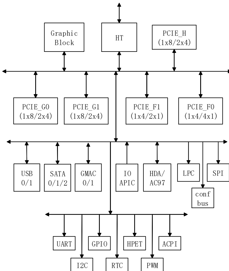
图 1-1. 桥片结构图
